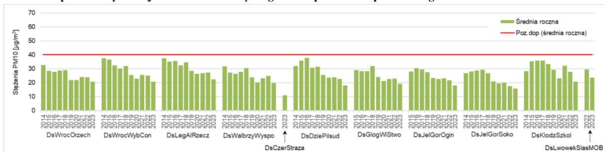
Wykres 1 Przebieg 36 maksymalnej wartości 24-godzinowej stężenia pyłu PM10 na poszczególnych stanowiskach pomiarowych województwa dolnośląskiego na tle poziomu dopuszczalnego w latach 1994 – 2023
