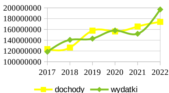
Wykres 1. Dynamika dochodów i wydatków Gminy w latach 2017-2022.
