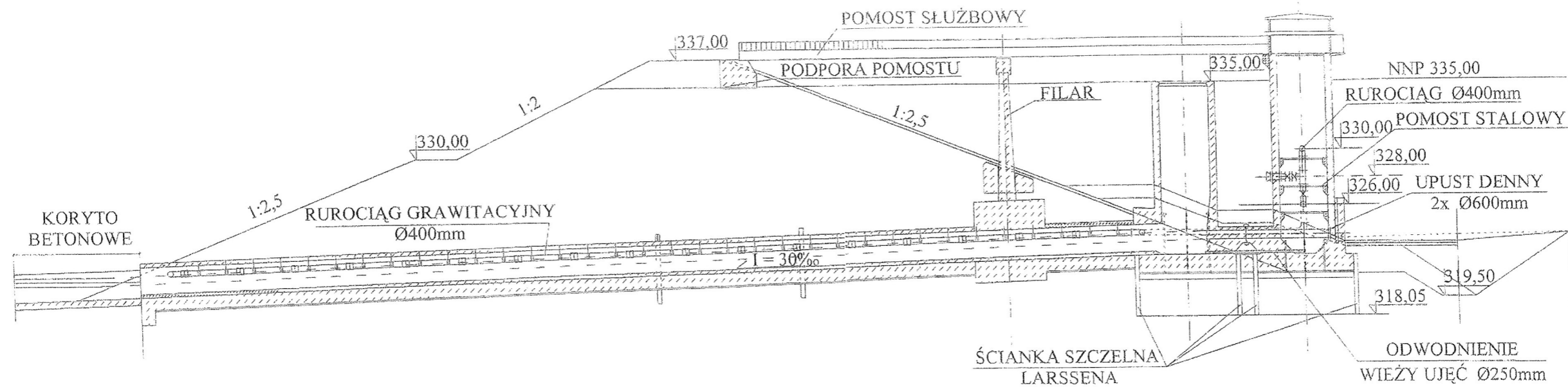
PRZEKRÓJ PODŁOŻNY PRZEZ BUDOWĘ PRZELEWOWO - UPUSTOWE WRAZ Z URZĄDZENIAMI TECHNOLOGICZNYMI
