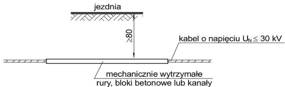
TABLICA SKRZYŻOWAŃ I ZBLIŻEŃ KABLI UŁOŻONYCH W ZIEMI DO INNYCH URZĄDZEŃ PODZIEMNYCH wg N SEP-E-004
