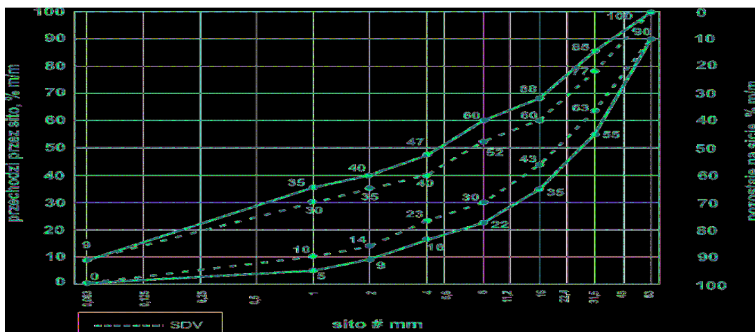
Rys. 6. Uziarnienie mieszanki niezwiązanej 0/63 dla podbudowy zasadniczej
