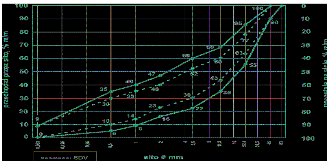
Rys. 5. Uziarnienie mieszanki niezwiązanej 0/45 dla podbudowy zasadniczej
